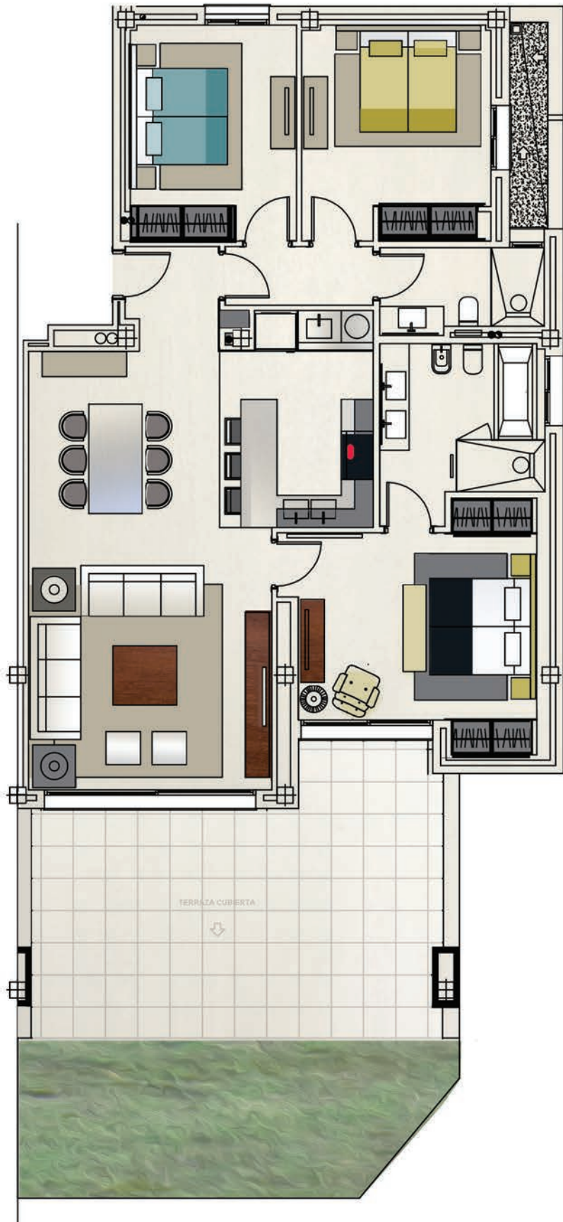
TIPO / TYPE A PLANTA BAJA / GROUND FLOOR 3 DORMITORIOS / BEDROOMS
